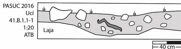
Figura 2.32c: Perfil de la unidad 41B1
