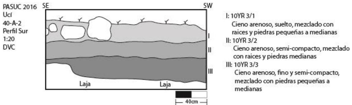
Figura 2.31d: Perfil de la unidad 40A2
