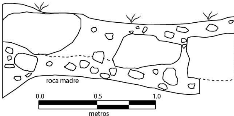
Figura 2.8c: Perfil este del pozo 17A2
