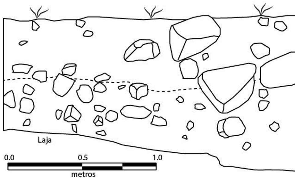
Figura 2.18b: Perfil sur del pozo 27A1.
