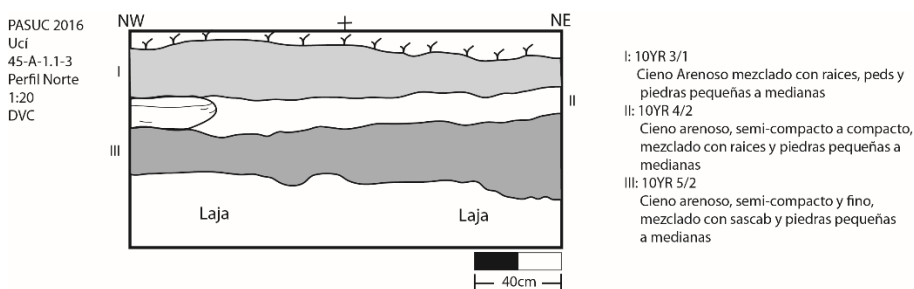
Figura 2.36b: Perfil de la unidad 45A1
