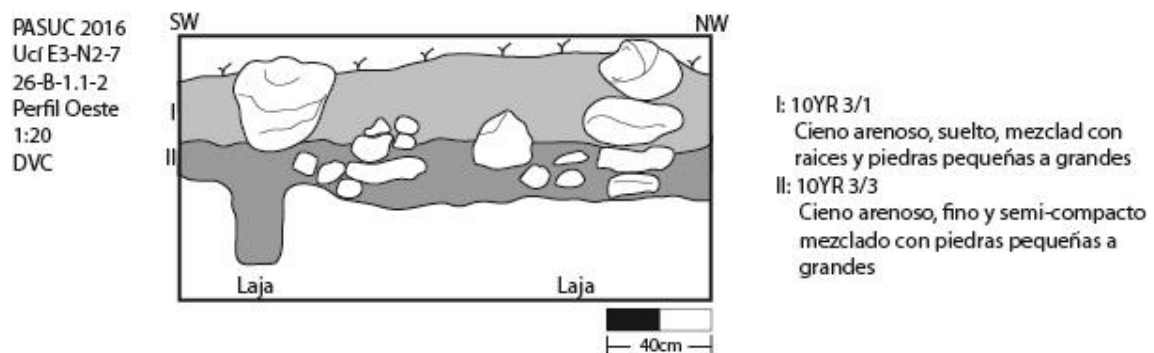
Figura 2.17c: Perfil de la unidad 26B1
