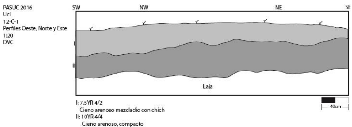
Figura 2.3g: Perfil de la unidad 12C1
