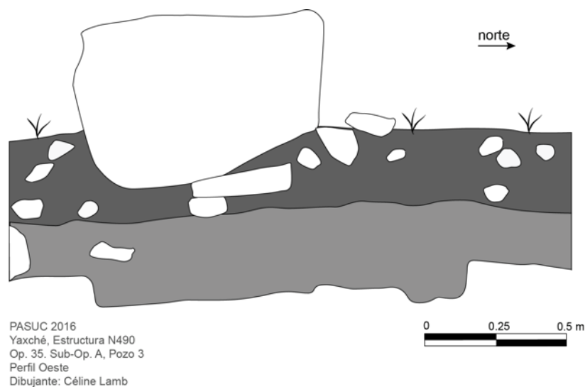
Figura 6.67: Perfil del pozo 35A3
