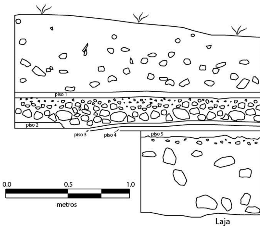
Figura 2.5c: Perfil sur de la unidad 14A2
