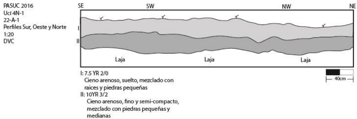
Figura 2.13c: Perfil de la unidad 22-A-1
