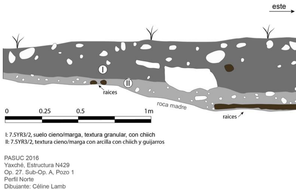
Figura 6.4: Perfil estratigráfico del pozo 27A1
