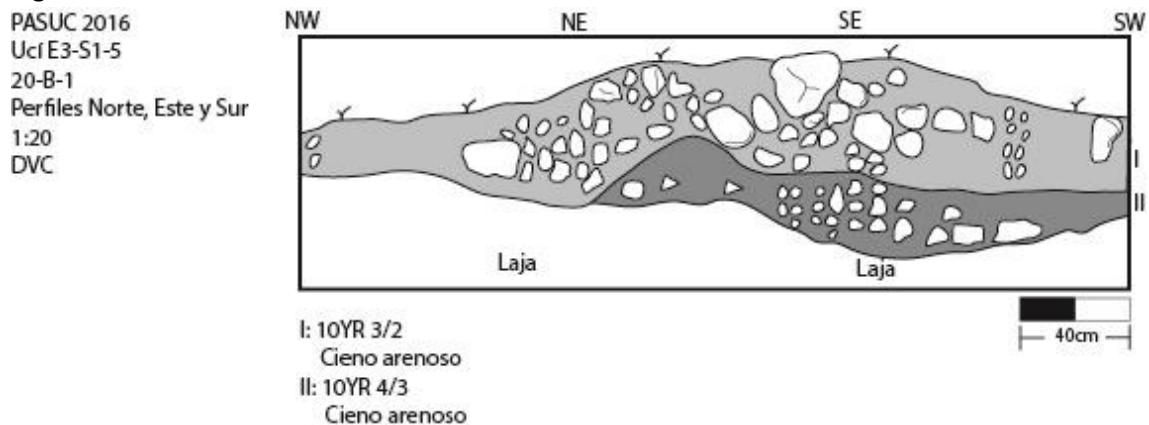
Figura 2.11d: Perfil de la unidad 20B1
