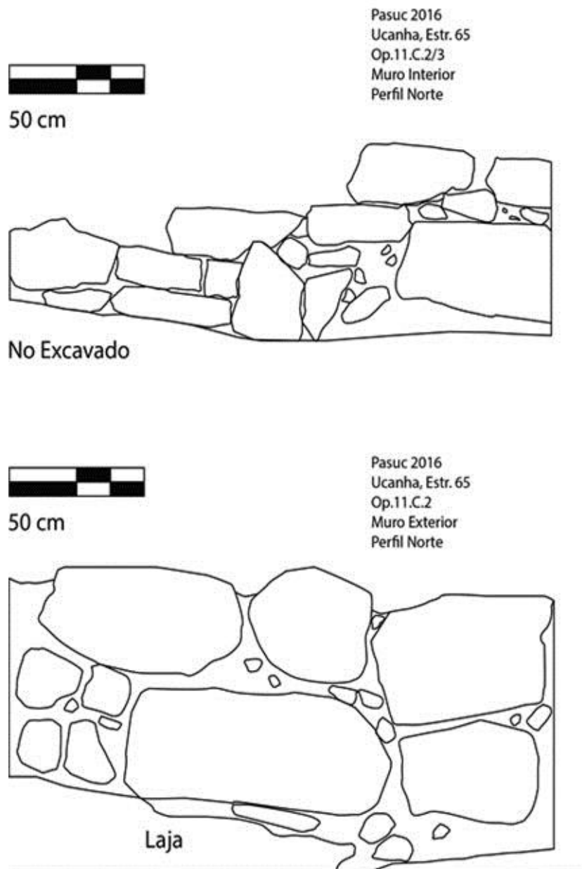
Figura 4.5. Perfiles nortes de los muros descubiertos en unidades C2 y C3.
