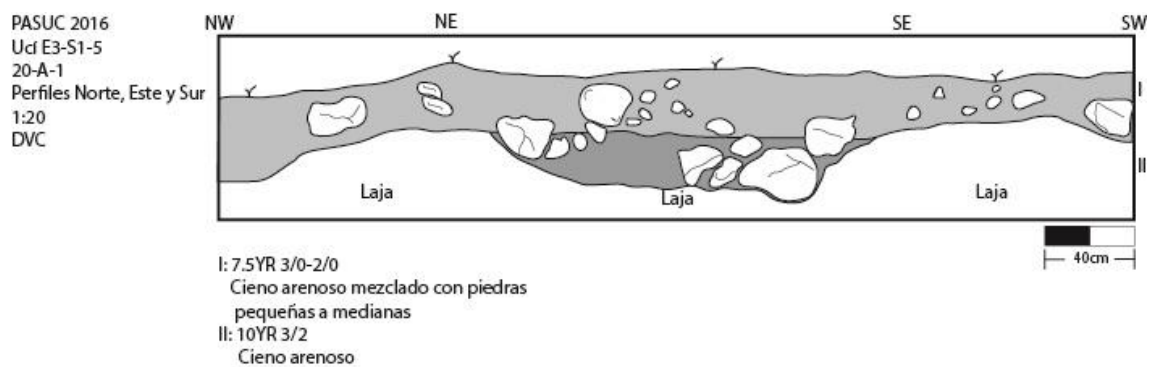
Figura 2.11b: Perfil de la unidad 20A1
