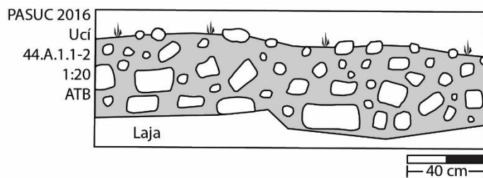
Figura 2.35b: Perfil de la unidad 44A1, lado norte
