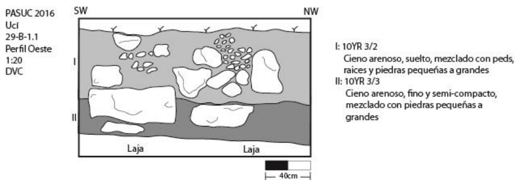
Figura 2.20e: Perfil de la unidad 29B1
