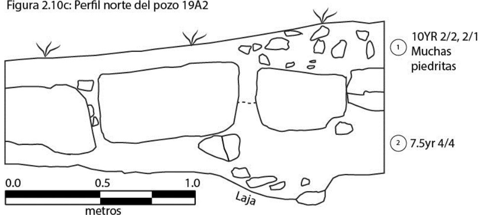
Figura 2.10c: Perfil norte del pozo 19A2
