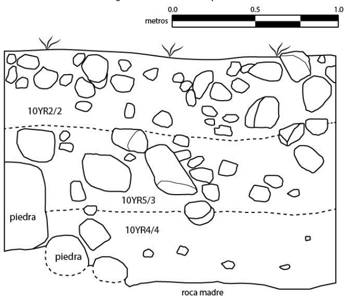
Figura 2.4b: Perfil sur del pozo 13A1.
