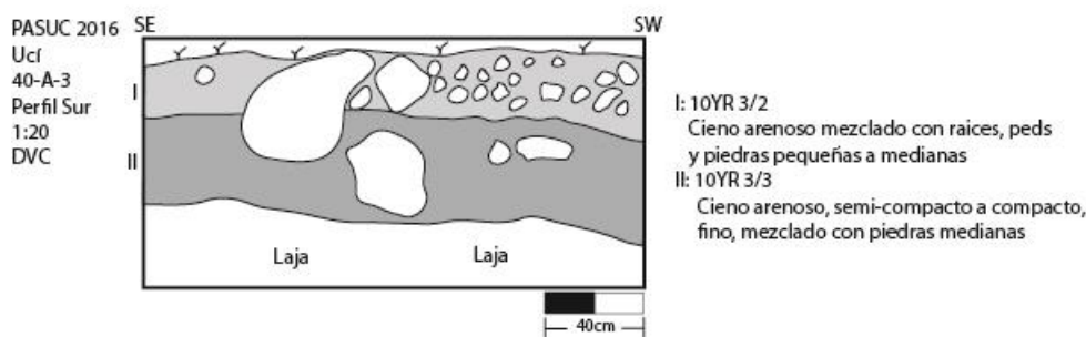
Figura 2.31g: Perfil de la unidad 40A3
