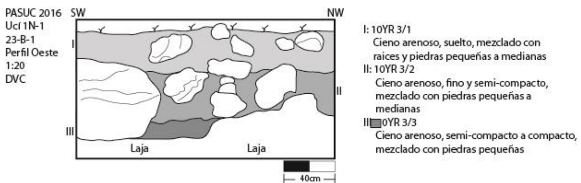
Figura 2.14e: Perfil de la unidad 23B1
