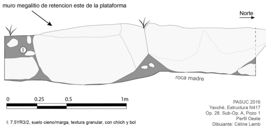
Figura 6.9: Perfil estratigráfico del pozo 28A1
