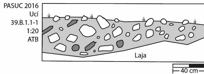
Figura 2.30c: Perfil de la unidad 39B1
