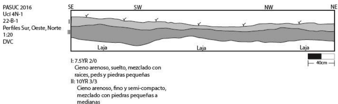
Figura 2.13e: Perfil de la unidad 22B1
