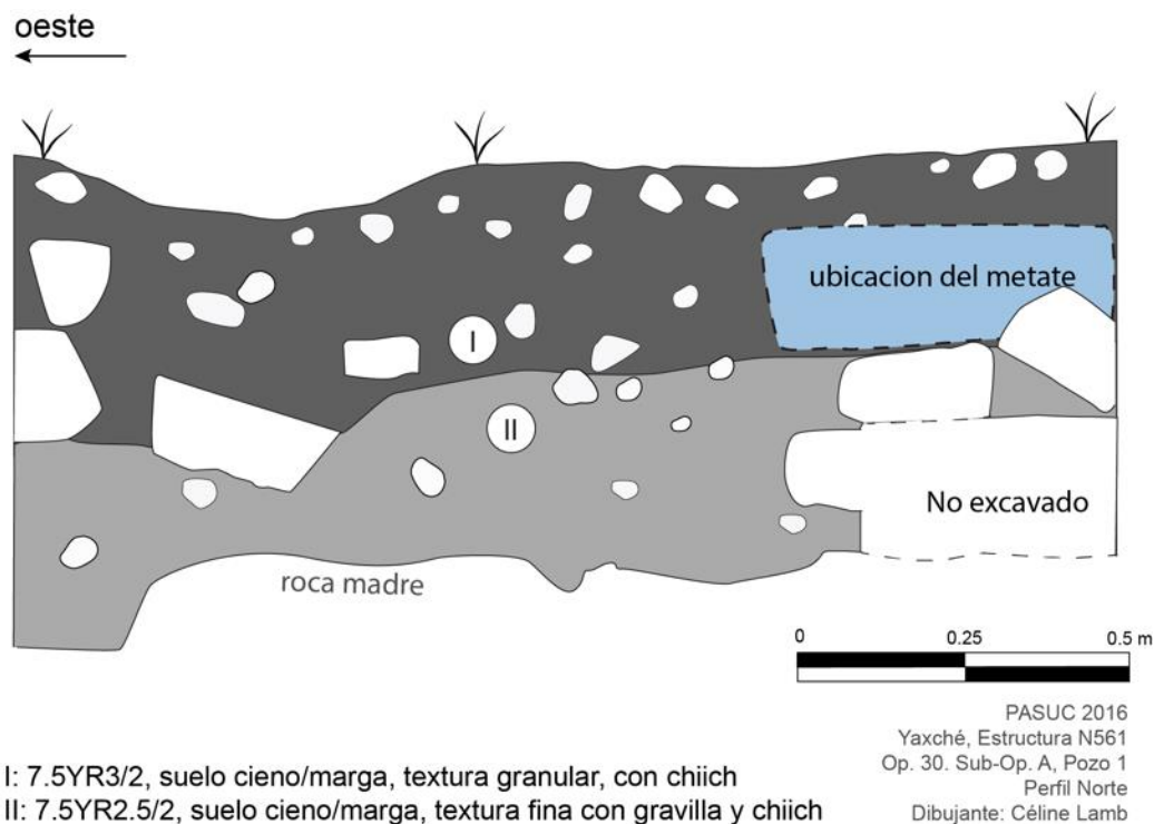
Figura 6.20: Perfil estratigráfico, pozo 30A1
