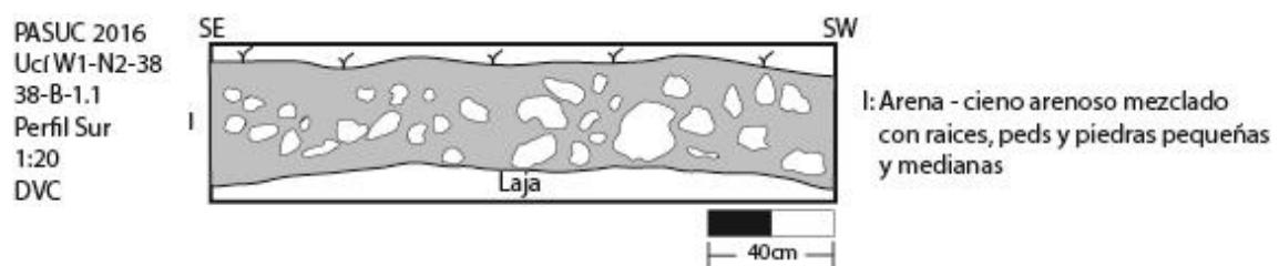
Figura 2.29f: Perfil de la unidad 38B1
