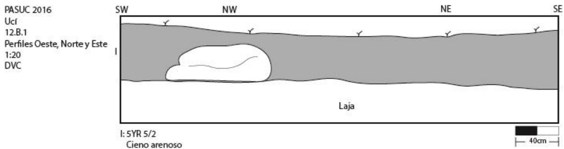
Figura 2.3d: Perfil de la unidad 12B1
