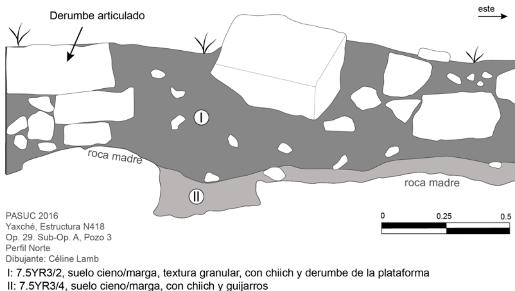
Figura 6.17: Perfil estratigráfico del Pozo 29A3
