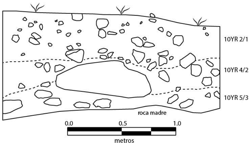
Figura 2.7c: Perfil oeste del pozo 16A2
