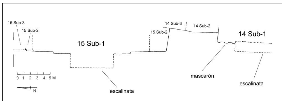
Figura 8 Planta de las fachadas oeste de los Edificio 14 y 15
