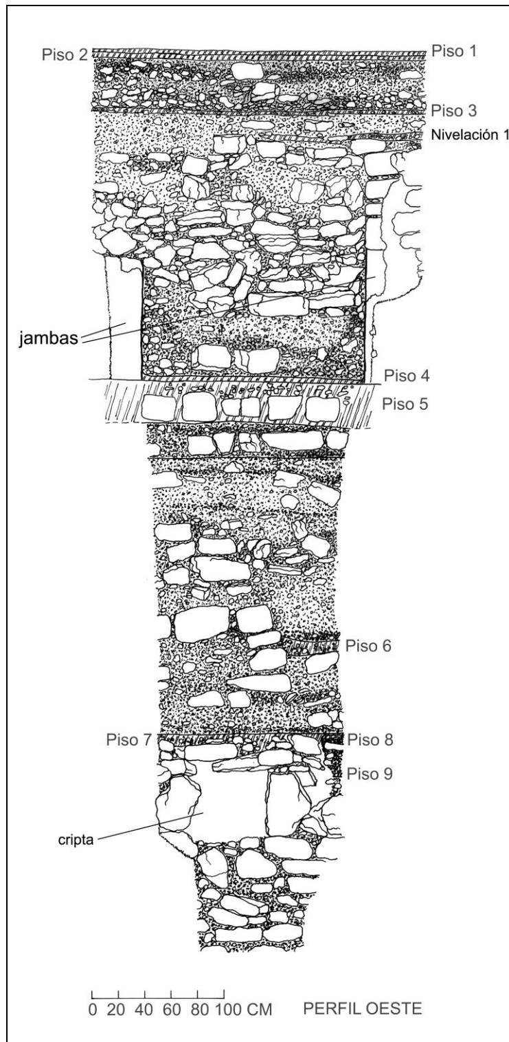
Figura 11 Dibujo del perfil oeste de la subop. 3A con la cripta protoclásica
