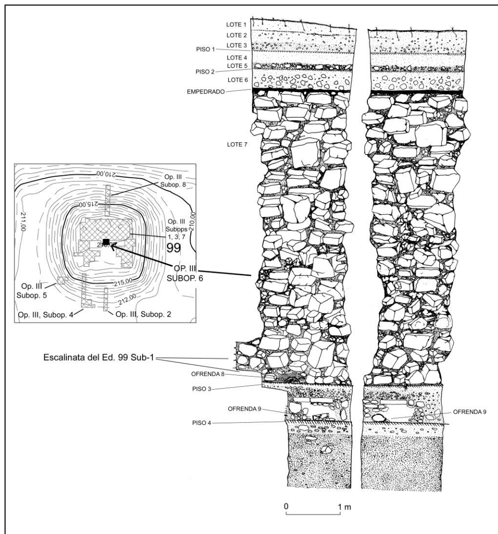
Figura 4 Perfil este y sur del pozo excavado en la parte superior del Edificio 99 (Op. III, Subop. 6) con ubicación de las Ofrendas 8 y 9 y subestructura del Edificio 99
