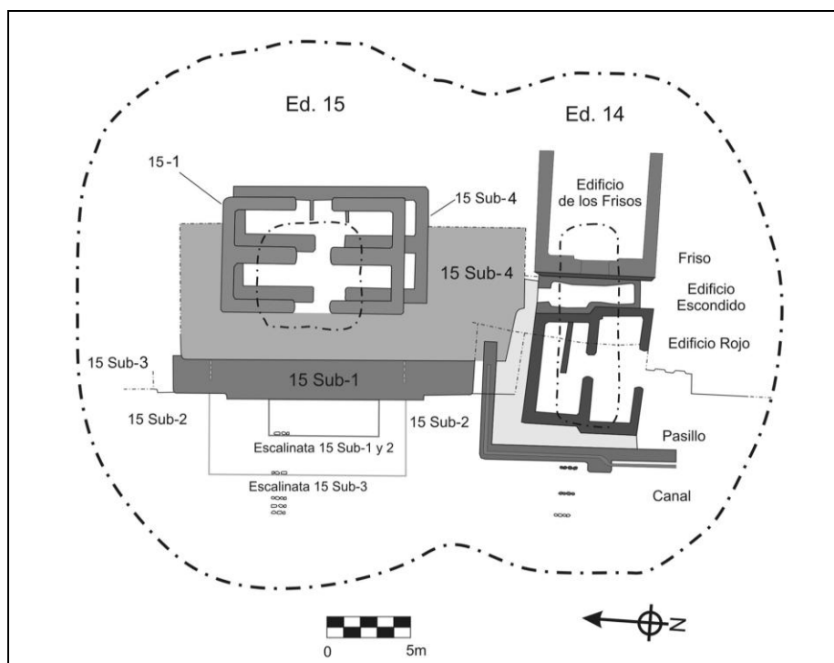
Figura 14 Planta de los Edificios 14 y 15
