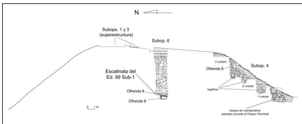
Figura 3 Corte N-S del Edificio 99 con ubicación de subestructura 99 Sub-1 y Ofrendas 8 y 9
