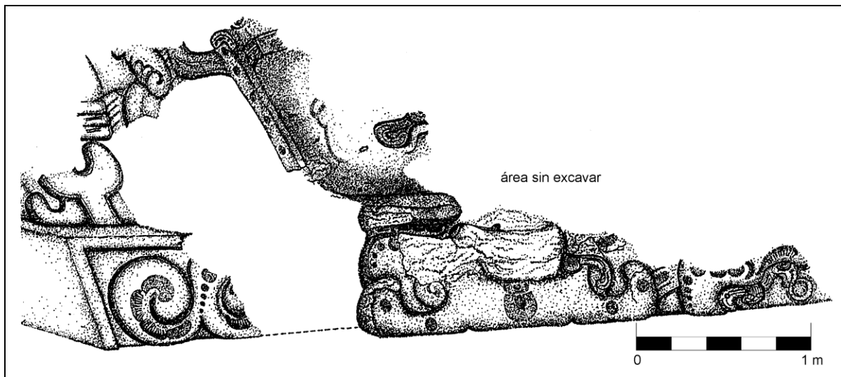
Figura 5 Isométrico de fachada edificio B-sub 2.
