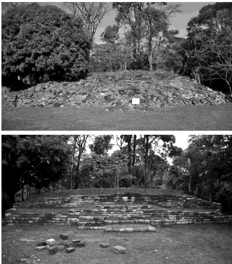
Figura 5 Estructura 34 antes y después de excavación y consolidación.
