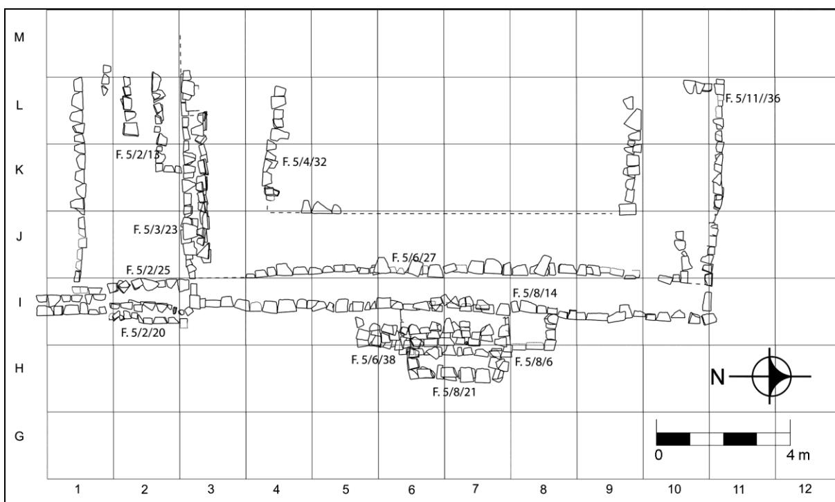
Figura 10 Estructura 34, Etapa VI.
