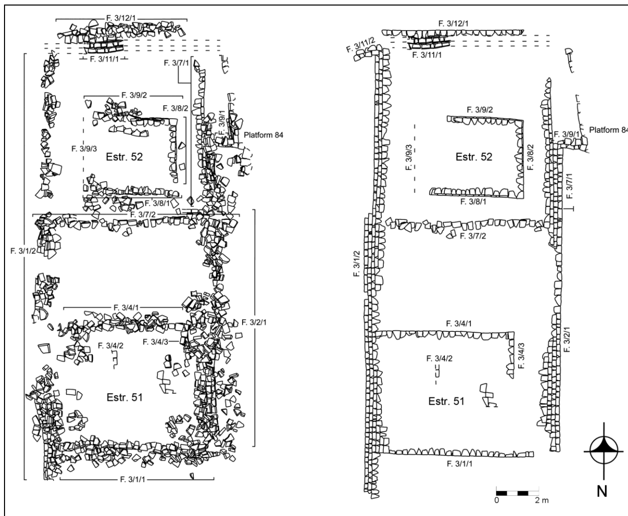
Figura 3 Estructura 51/52 antes y después de excavación y consolidación.
