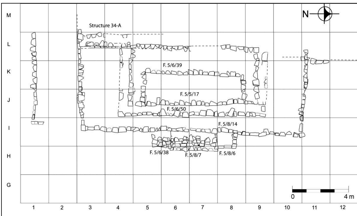
Figura 8 Estructura 34, Etapa IVc.
