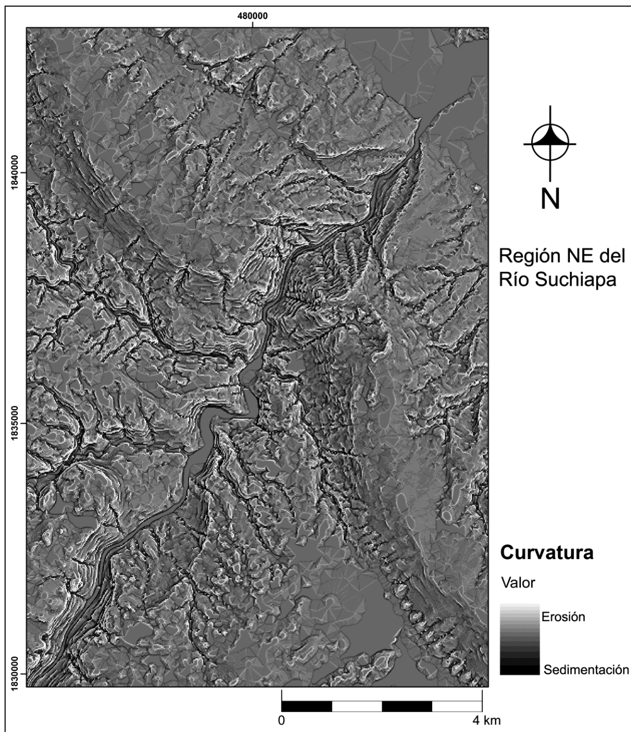
Figura 5 Análisis de curvatura: G. Acosta, E. Méndez, V. García, I. Ozuna (Datum UTM WGS84).
