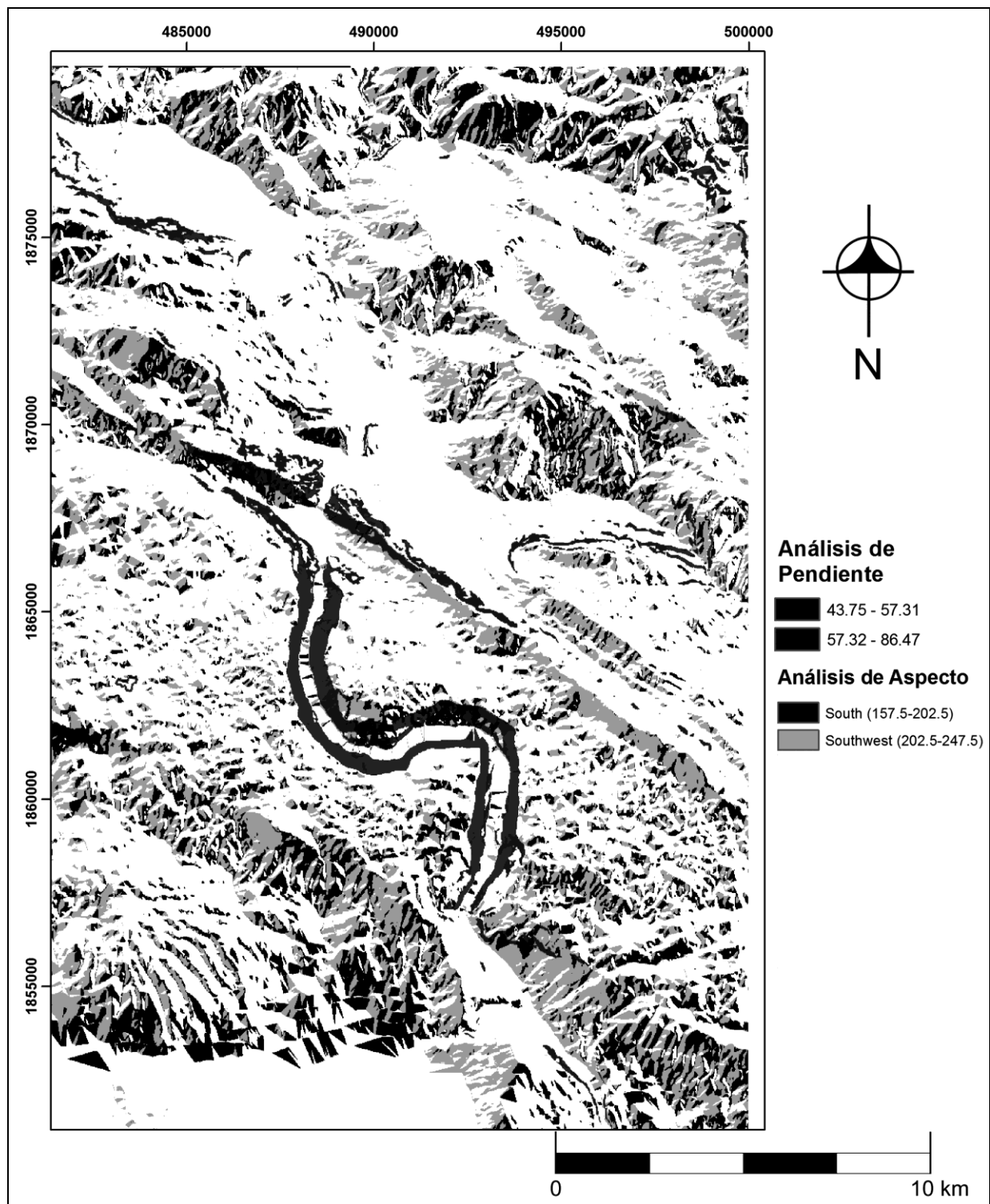
Figura 4 Análisis de Pendiente-Aspecto: G. Acosta, E. Méndez, V. García, I. Ozuna (Datum UTM WGS84).
