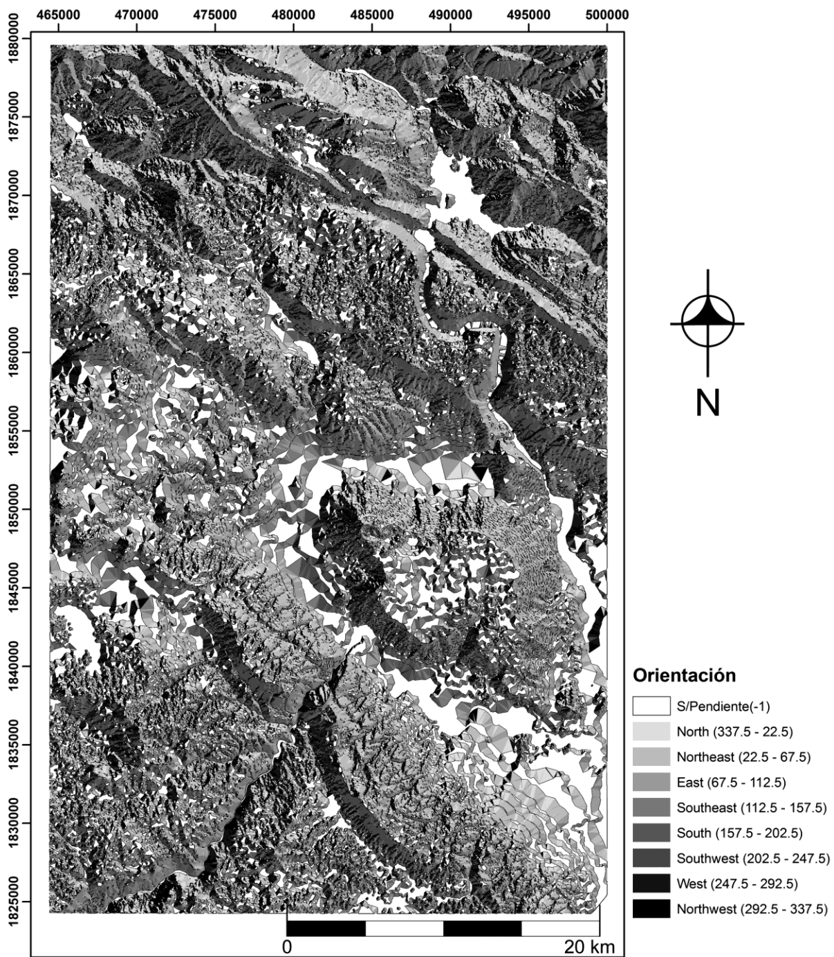
Figura 3 Análisis de aspecto u orientación.
