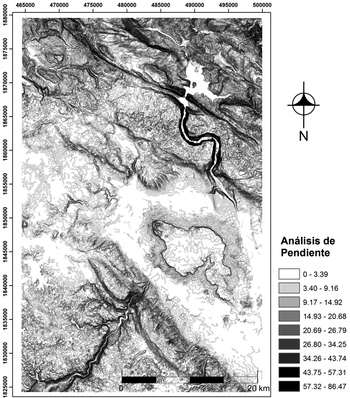
Figura 2 Análisis de pendiente: G. Acosta, E. Méndez, V. García, I. Ozuna (Datum UTM WGS84).
