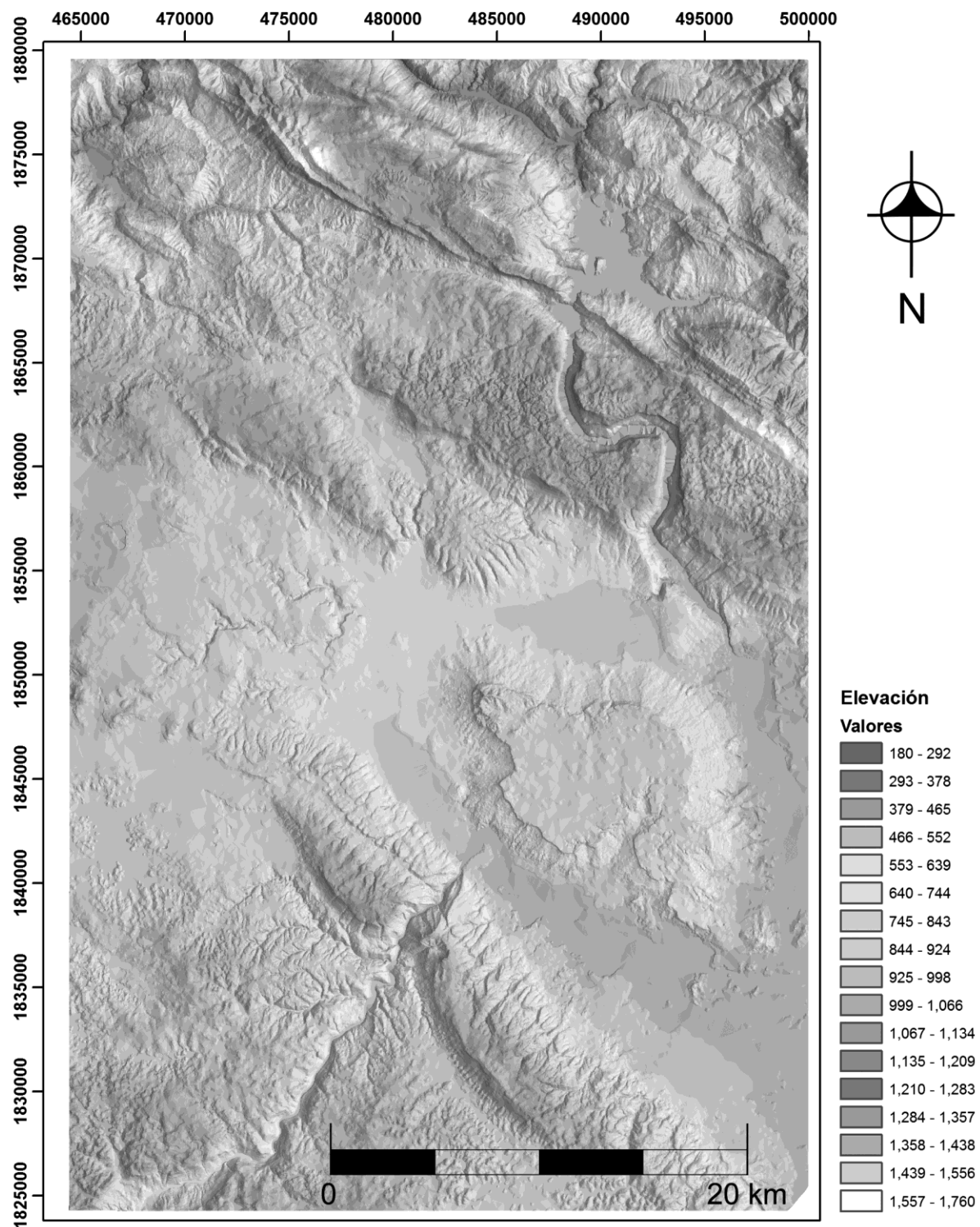
Figura 1 Modelo digital de elevación: G. Acosta, E. Méndez, V. García, I. Ozuna (Datum UTM WGS84).
