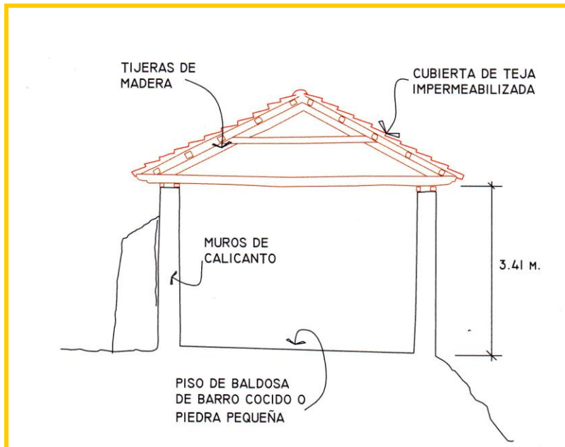
Figura 4 Dibujo en Sección, Ermita del Soldado, San Juan Chamelco, Alta Verapaz. Dibujó Víctor Sandoval; Digitó Jorge Cáceres
