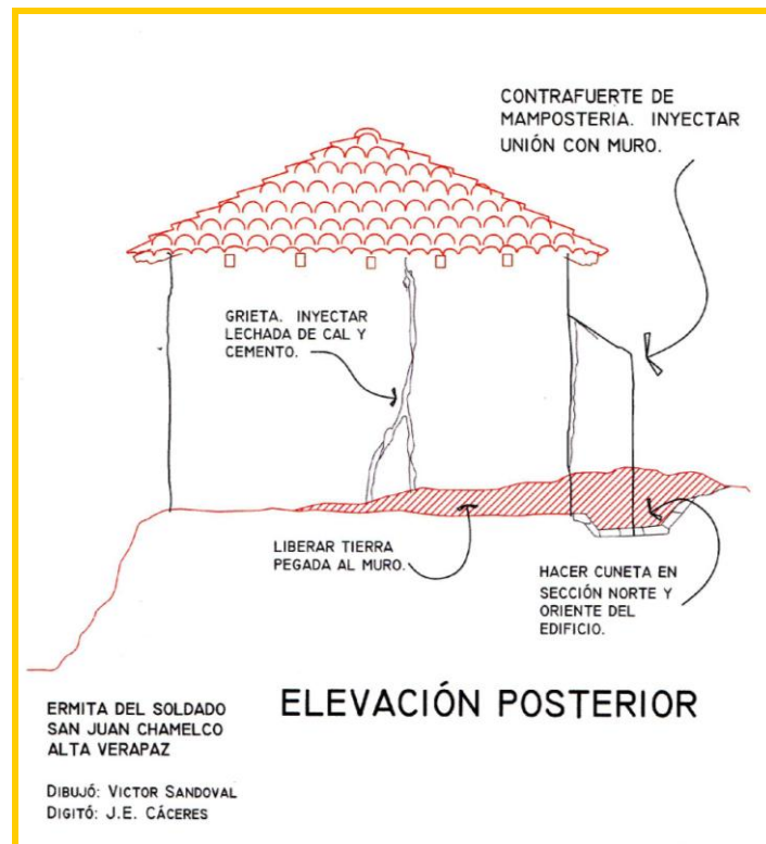
Figura 5 Dibujo de Ermita del Soldado. Procedimiento de Restauración
