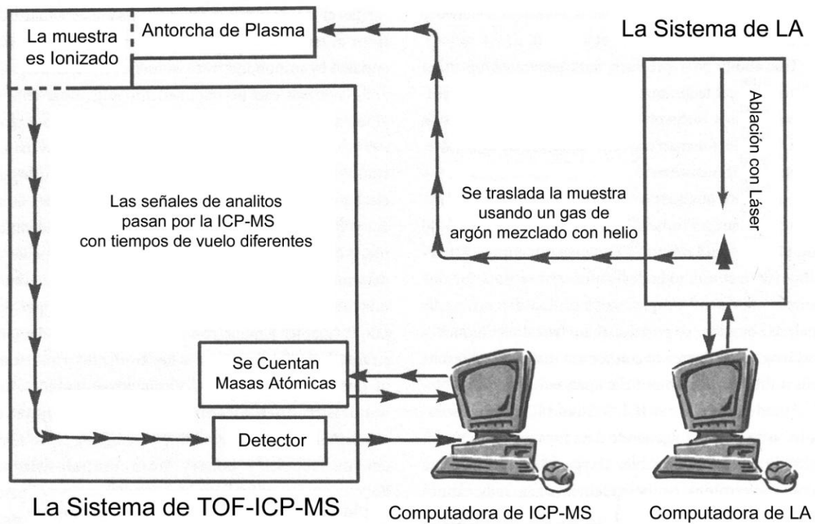
Figura 1 Diagrama de los sistemas de LA-TOF-ICP-MS (después de Speakman y Neff 2005:5)
