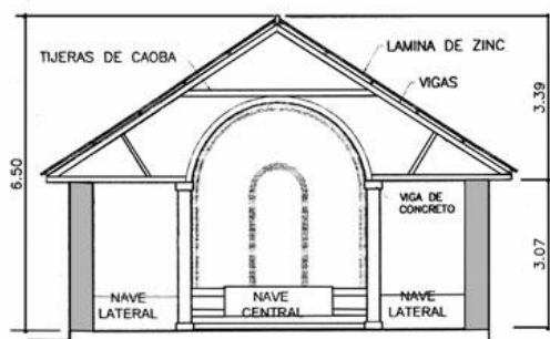
Figura 8 Secciones
