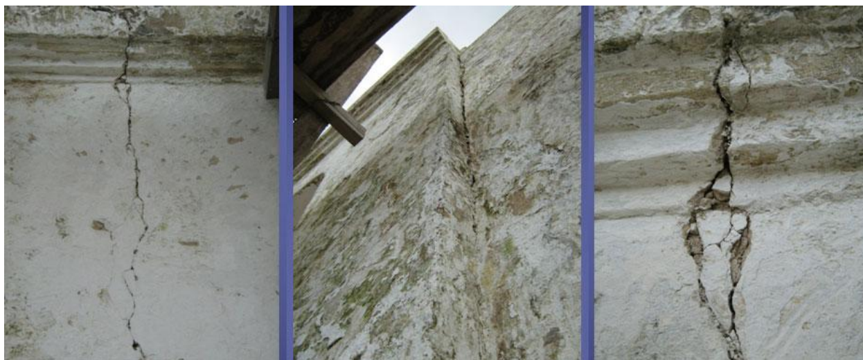
Figura 19 Grietas expuestas
