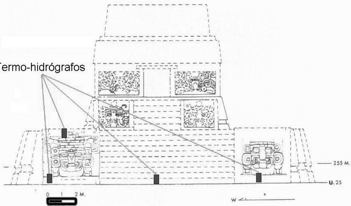
Figura 2 Localización de Termo-hidrógrafos Estructura 5D-33 sub 3
